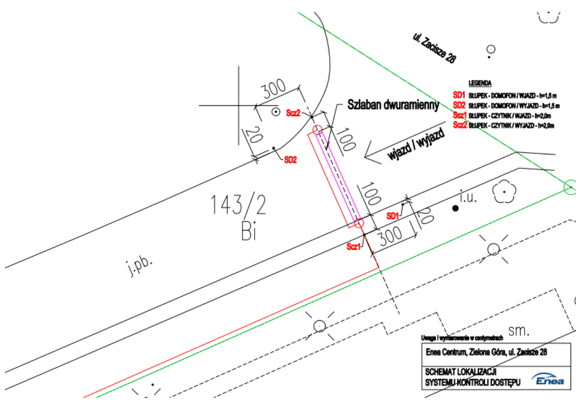
Rysunek nr 1 – panele wywoławcze do wideodomofonów przy szlabanie
