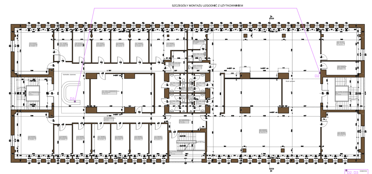
Rysunek nr 3 – rzut 1 piętra – lokalizacja paneli odbiorczych ( 2 sztuki )
